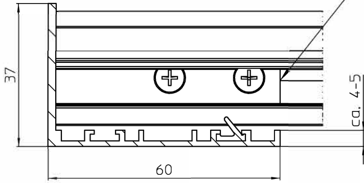
Schnitt Seitenabschluss Maßstab 1:1
